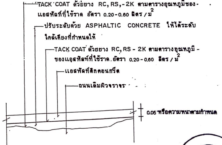
รายละเอียดงาน OVERLAY ด้วย ASPHALTIC CONCRETE not to scale
