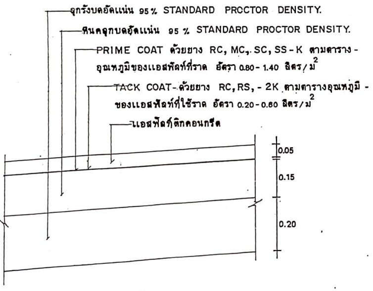
รายละเอียด ASPHALTIC CONCRETE not to scale
